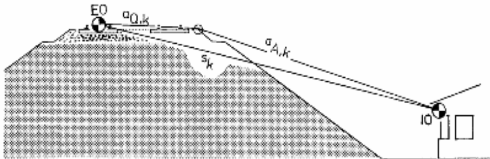
Bild 4: Größen zur Berechnung des Schirmwertes an einem Damm
