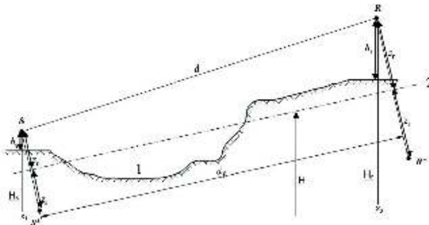
Abbildung 5.2: Äquivalente Höhen über der Mittleren Grundlinie
