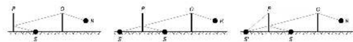
Abbildung 5.8: Konstruktion des fiktiven gebeugten Ausbreitungswegs mit der Oberkante des Reflektors als Beugungspunkt unter homogenen Ausbreitungsbedingungen
