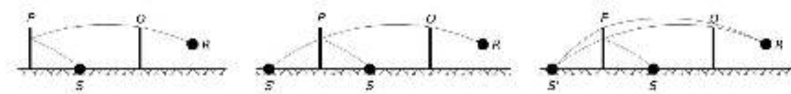
Abbildung 5.9: Konstruktion des fiktiven gebeugten Ausbreitungswegs mit der Oberkante des Reflektors als Beugungspunkt unter günstigen Ausbreitungsbedingungen
